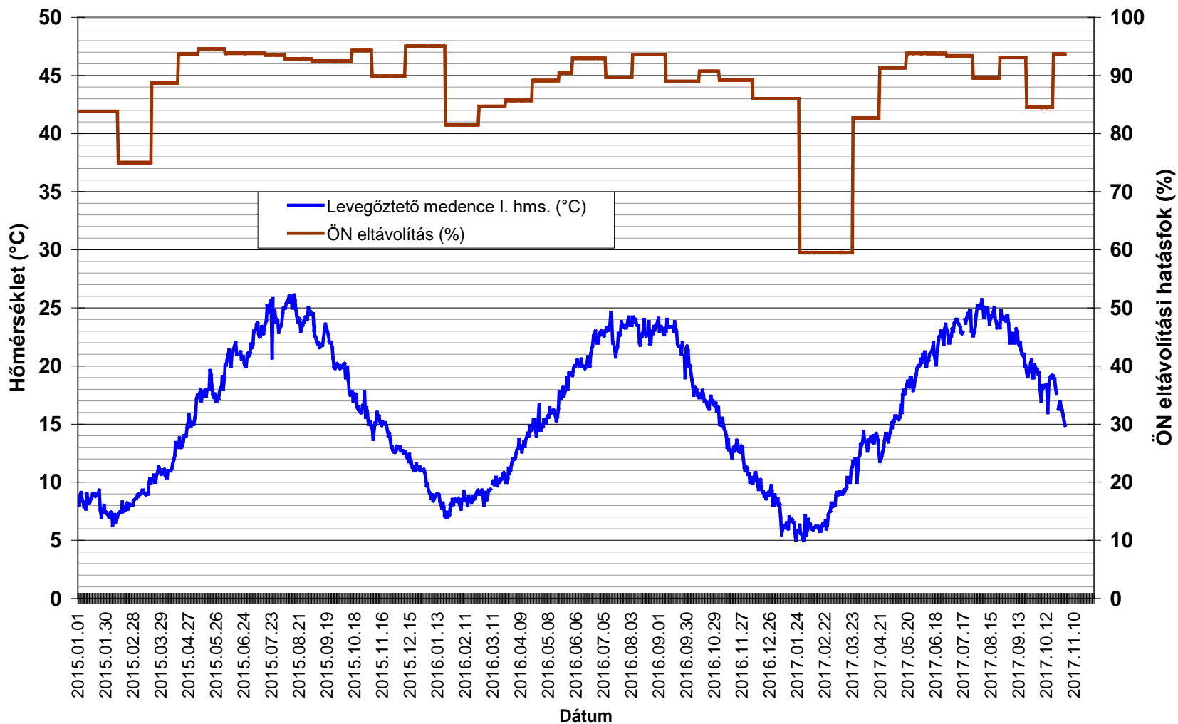
Levegőztető medence vízhőmérséklet - ÖN eltávolítási hatások idősor
