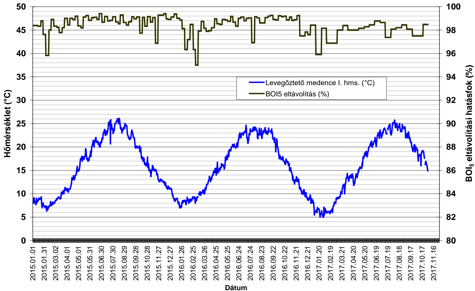
Levegőztető medence vízhőmérséklet - BOI_5 eltávolítási hatások idősor
