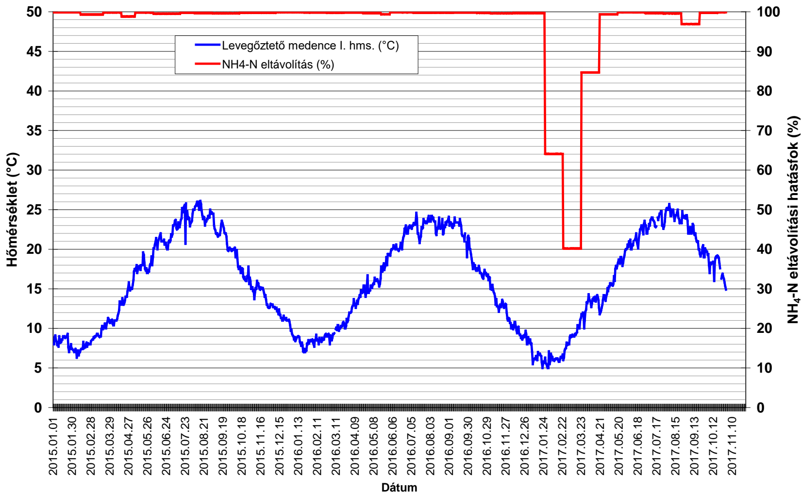
Levegőztető medence vízhőmérséklet - NH 4 -N eltávolítási hatások idősor
